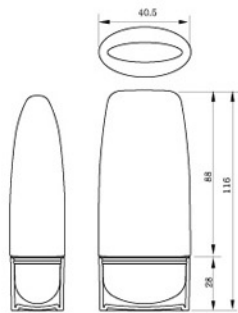
GLP SU-60 • MAT'L : PP, EVOH, PN-200 • 60ml
