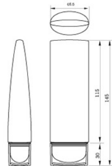
GLP STS-70 • MAT'L : PN22, PP, EVOH • 70ml
