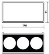
GLP PR-7 • MAT'L : ABS, EVA
