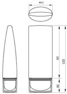
GLP STS-60 • MAT'L : PN22, PP, EVOH • 60ml
